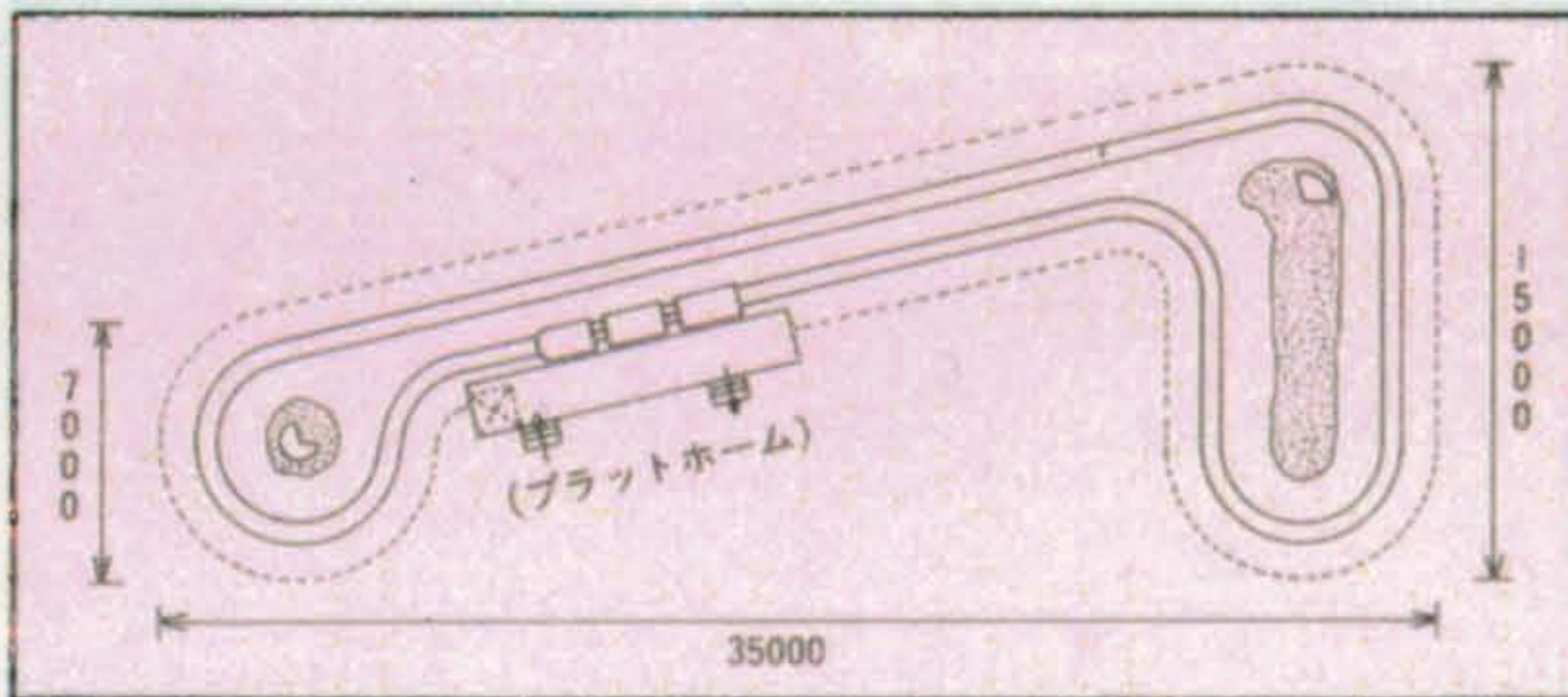
■「みさき公園」のレールレイアウト例(レール長約88m)
